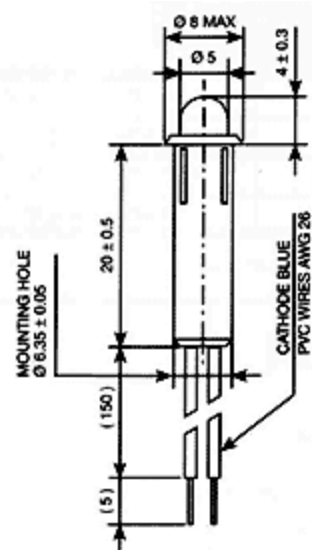
MD-577X
