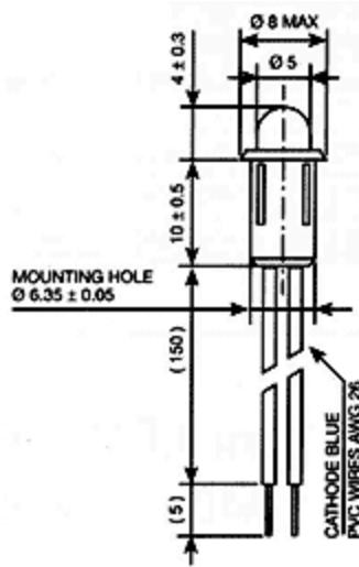
MD-567X
